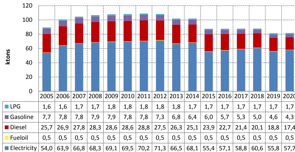
Διάγραμμα 3.39. ΝΣΔΑΕ σενάριο – Προβολή πρωτογενούς ζήτησης ενέργειας ανά ενεργειακό φορέα
