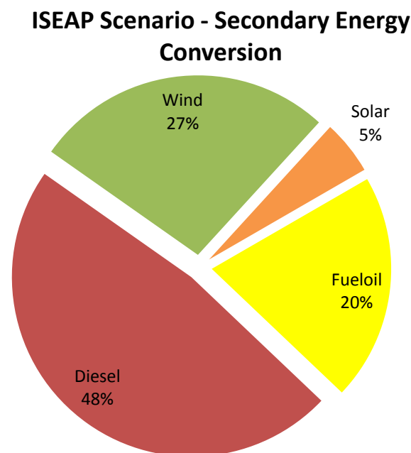
Διάγραμμα 3.36. ΝΣΔΑΕ σενάριο – Δευτερογενής μετατροπή ενέργειας το 2020
